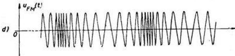
Slika: a) Nosilac; b) modulišuci signal; c) fazno modulisan signal; d) frekvencijski modulisan signal
